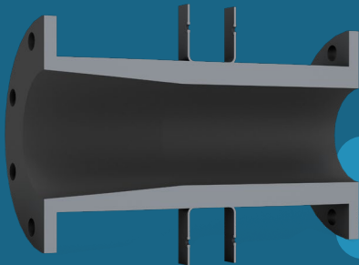
Manga Cone Aplicaciones Modulantes Altamente Abrasivas
