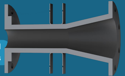
Manga Cone Funnel Aplicaciones Modulantes
